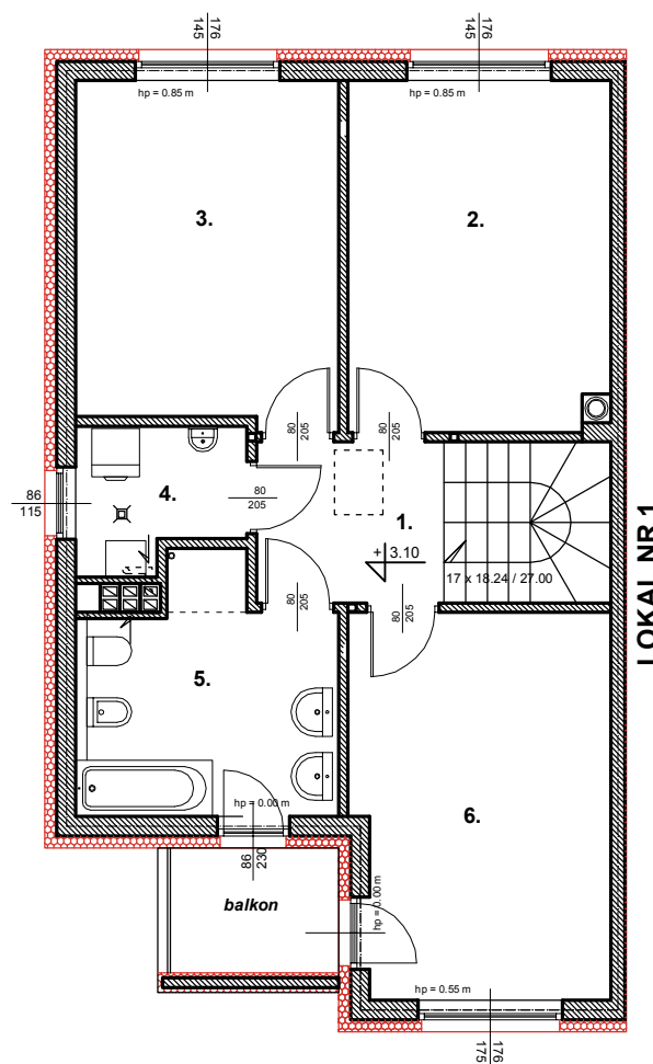
RZUT PIĘTRA BUDYNEK NR 3, LOKAL NR 2, ul. Nowowiejska 32B/2
