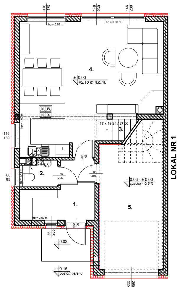
RZUT PARTERU BUDYNEK NR 3, LOKAL NR 2, ul. Nowowiejska 32B/2
